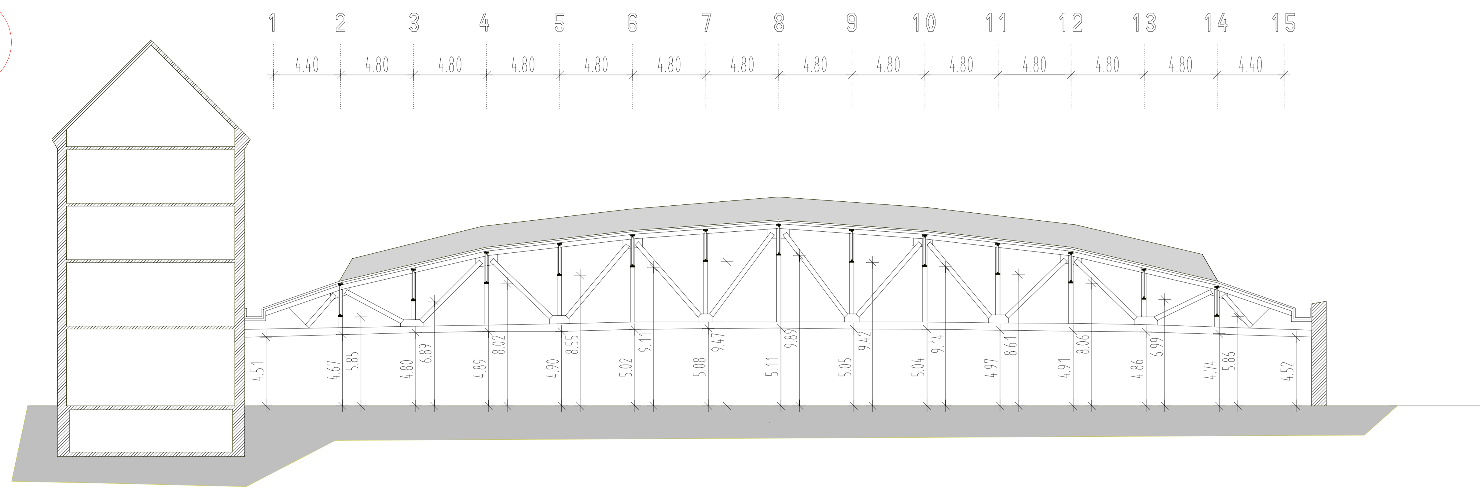
Verwaltungsgebäude Halle (Träger 1: Glashausseite) Spreeseite
