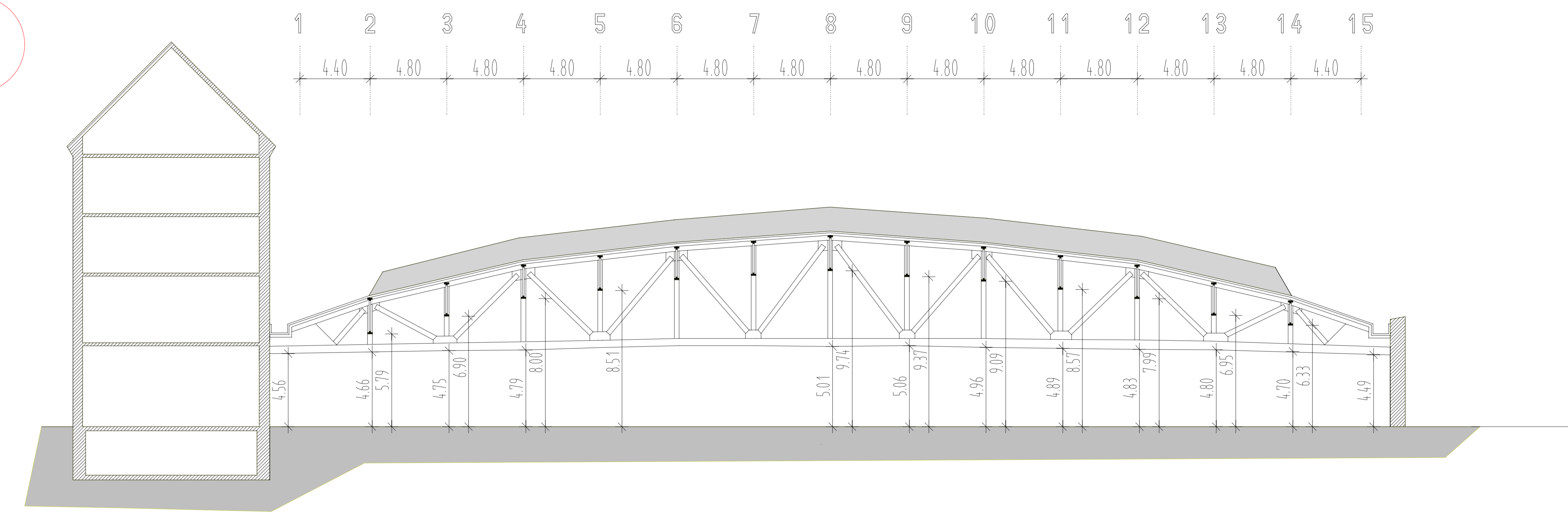
Verwaltungsgebäude Halle Spreeseite
