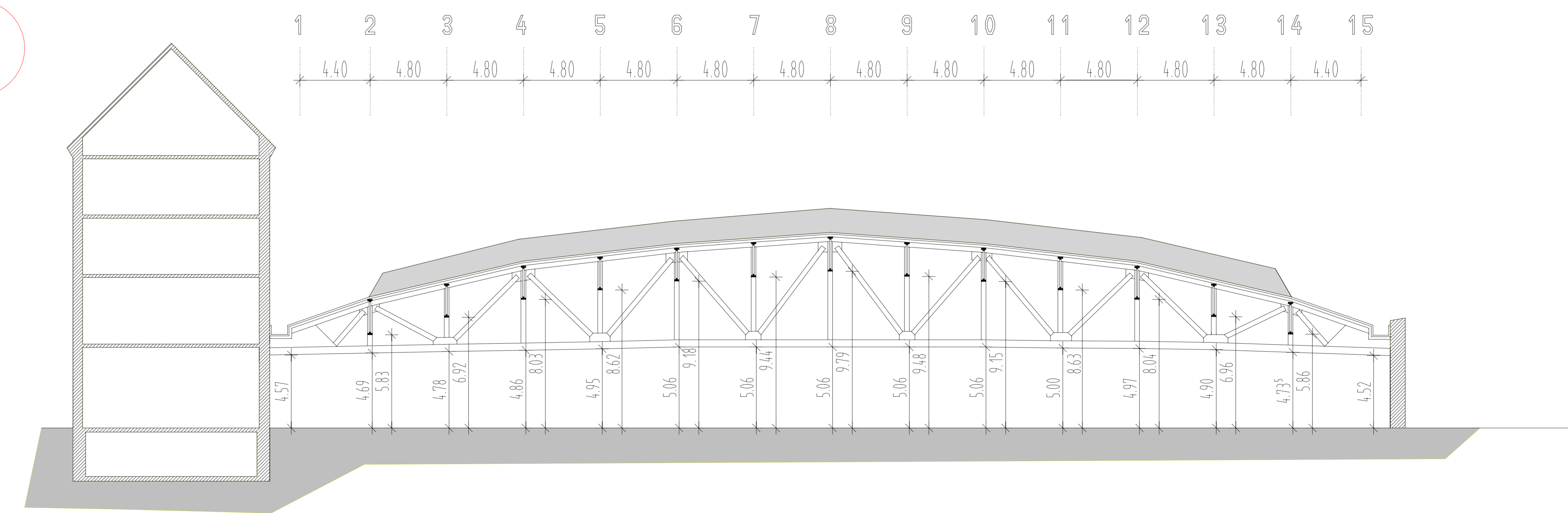
Verwaltungsgebäude Halle (Träger 4: Straßenseite Eichenstraße) Spreeseite
